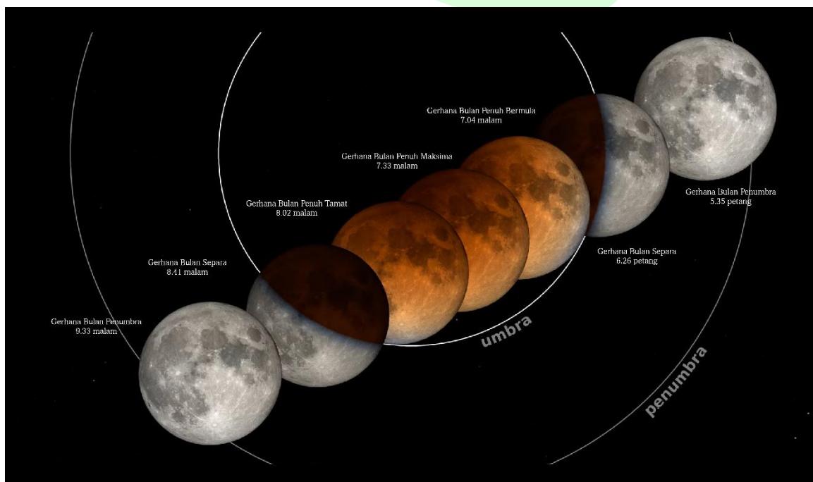
Rajah 2: Keadaan Bulan ketika masuk bayang Penumbra dan Umbra pada 3 Mac 2026 (Selasa)
