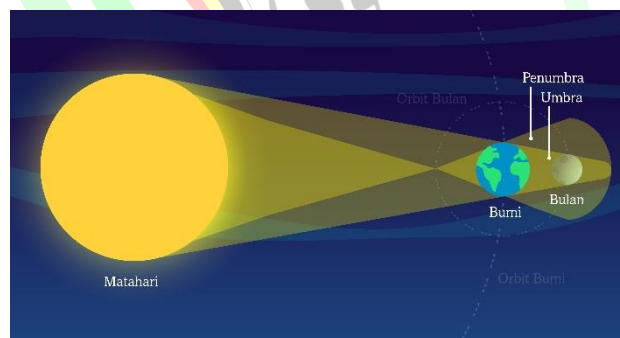
Rajah 1: Kedudukan Matahari, Bumi dan Bulan ketika Gerhana Bulan
